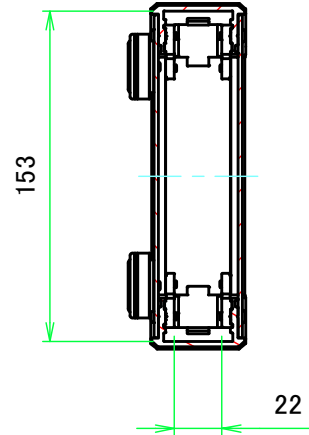
A-A (1 : 3.5)
