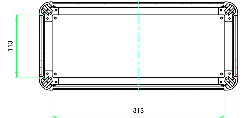
C-C (1 : 3.5)
